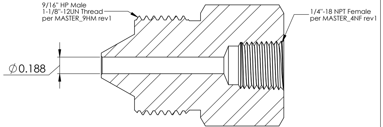
SECTION A-A SCALE 1.5 : 1
